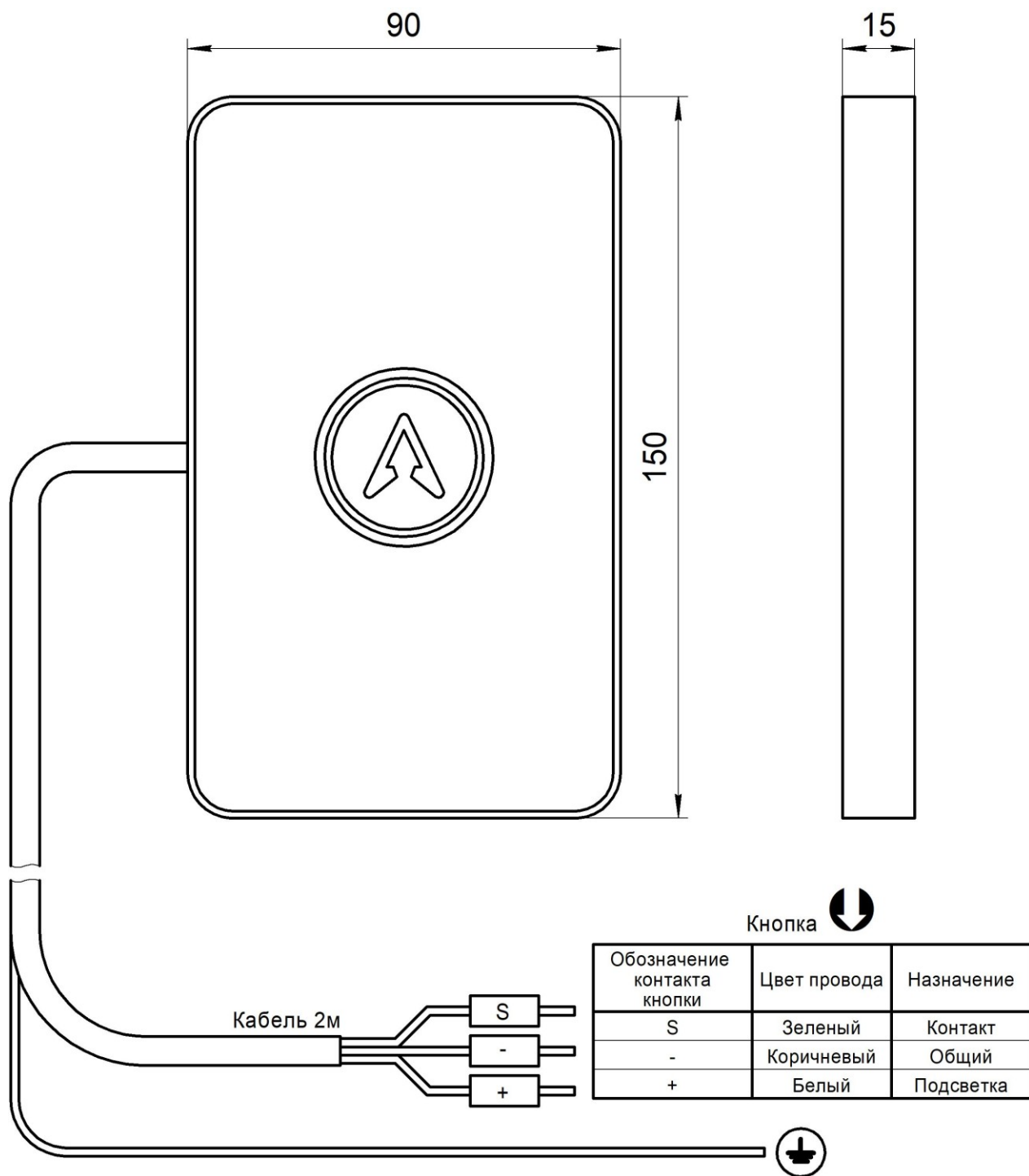
Рис.1 Внешний вид и габаритные размеры Вызывного поста ОНИКС НШЕК.468381.124-01
